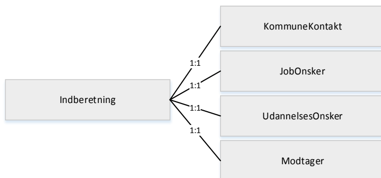
Figur 1 XML struktur for afhentning af hændelser
