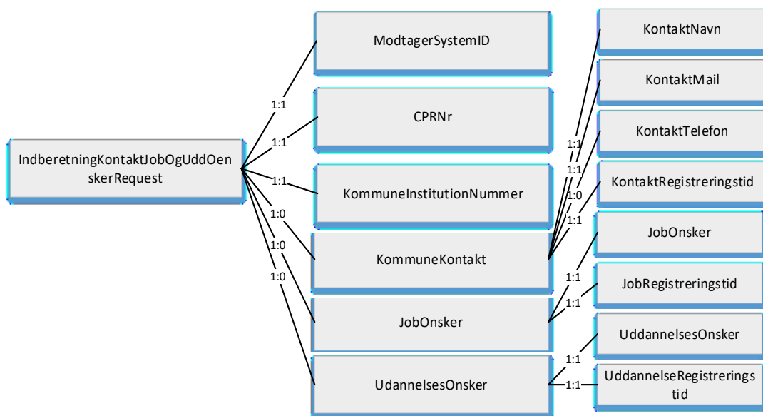
Figur 4.1 XML struktur for Indberetning af kontaktoplysninger, uddannelsesønsker og jobønsker fra kommunen
